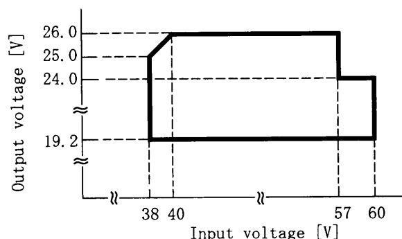
Fig. 2.1 Input voltage derating curve 入力電圧デレティング
