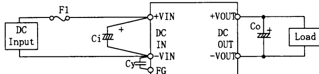
Fig. 2.2 External components 外付け部品
