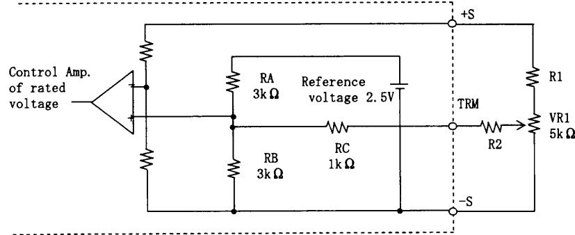
Fig. 2.5 Output voltage control circuit 出力電圧制御回路
