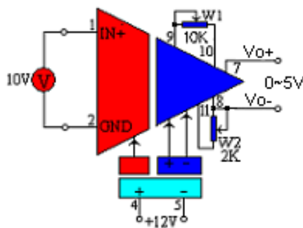
0~5V 电压输出型典型接线参考图
