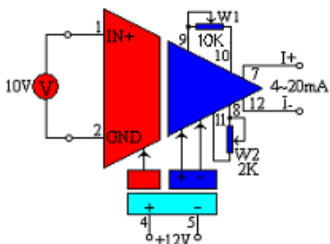
4~20mA 电流输出型典型接线参考图
