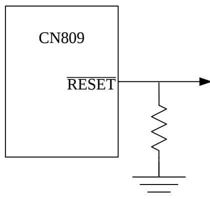
图4 V_{CC}=0V 时复位信号有效
