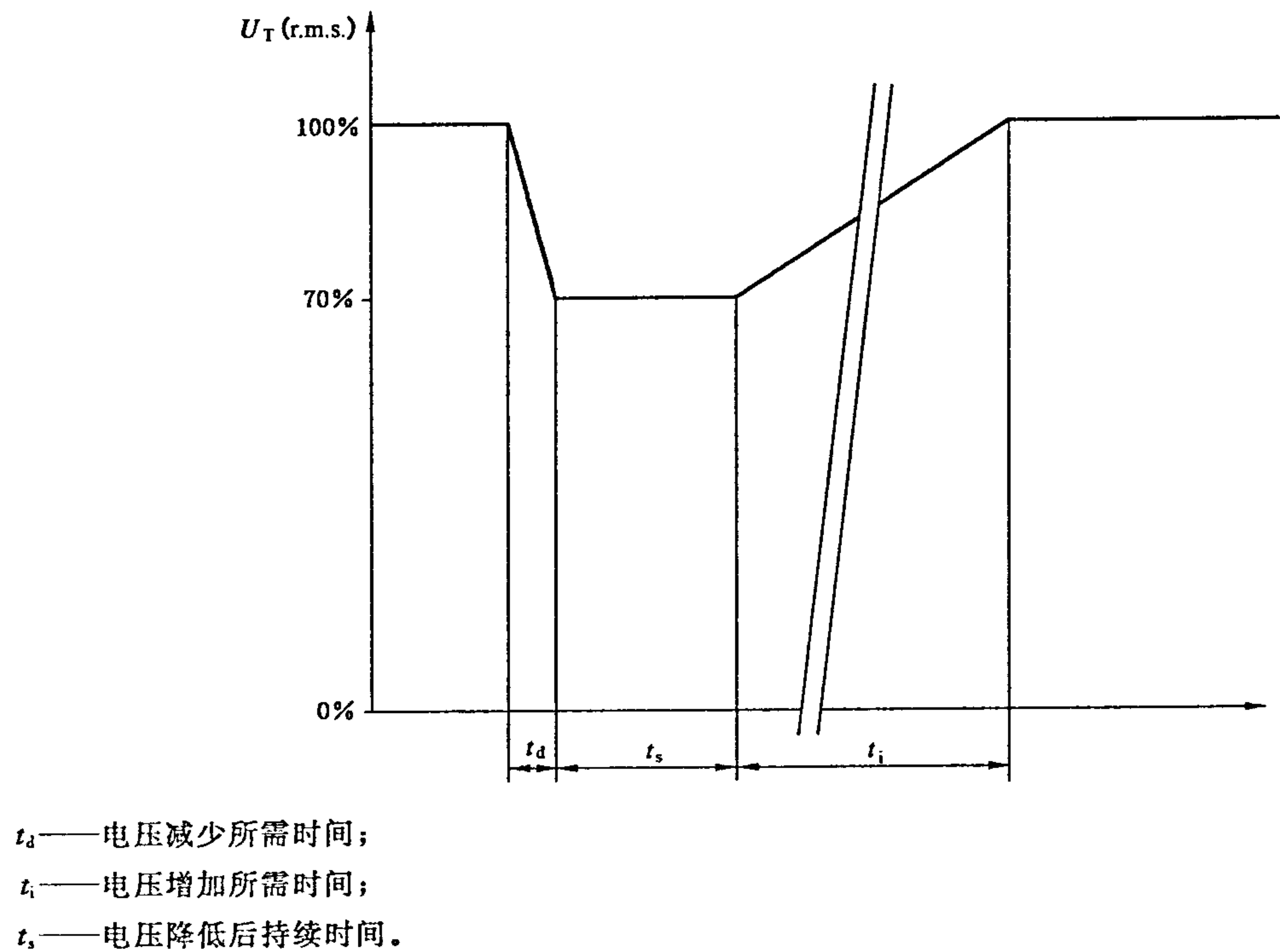
图 3 电压变化
