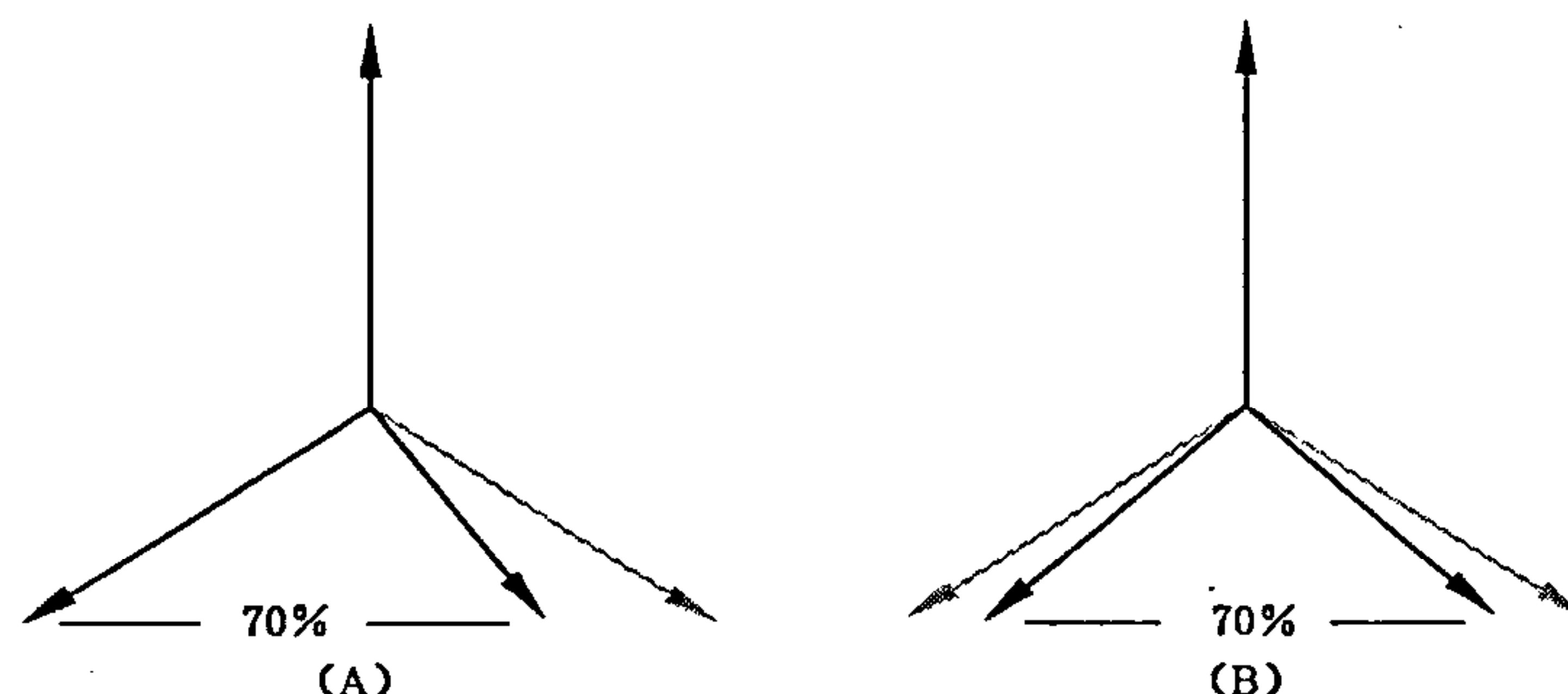
a) 三相系统的相线对中线试验
