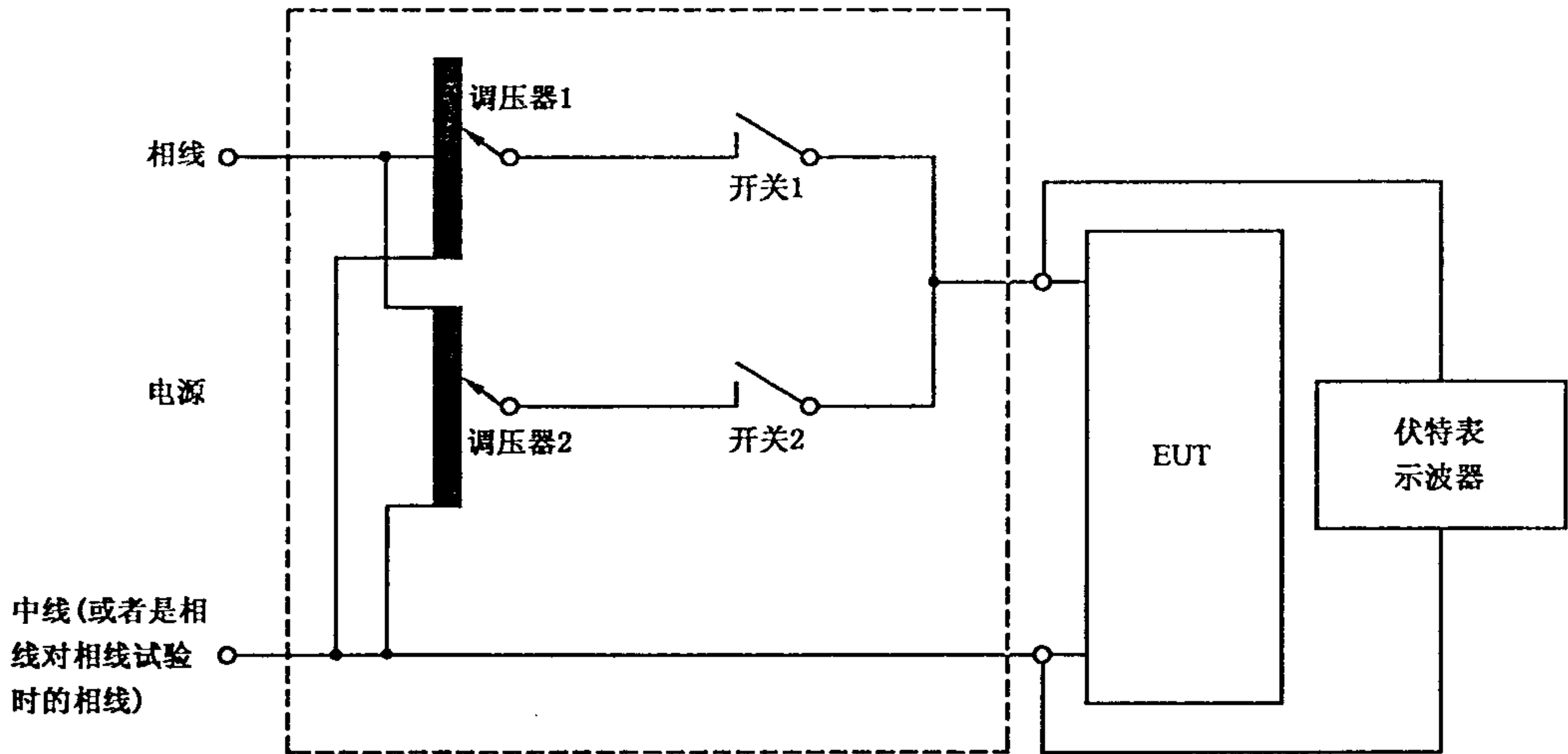
a) 采用调压器和开关进行电压暂降、短时中断和电压变化的试验原理图
