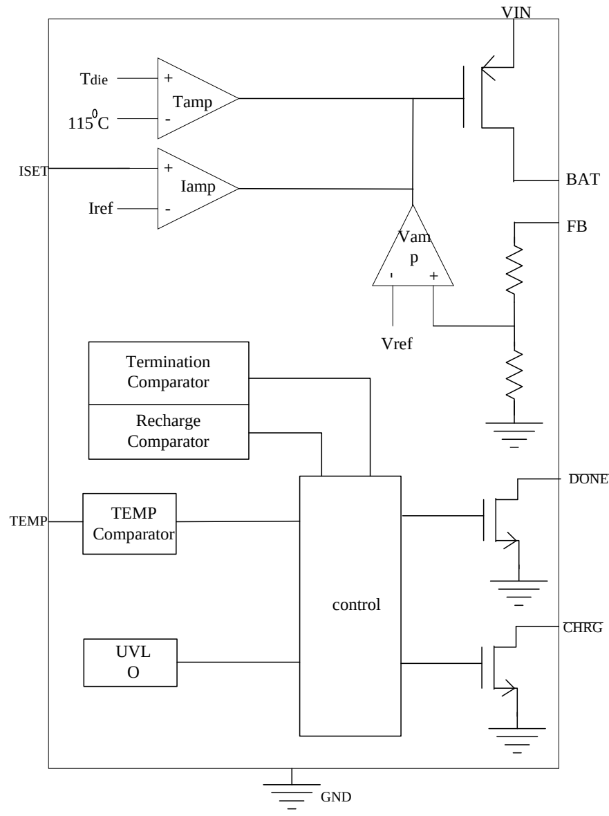
图 3 功能框图
