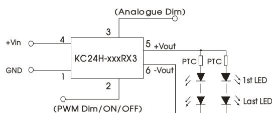
图 3 串并联应用
