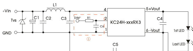
图 5 EMC 推荐电路
