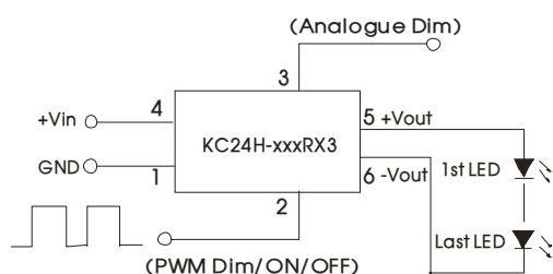
图 2 串联应用
